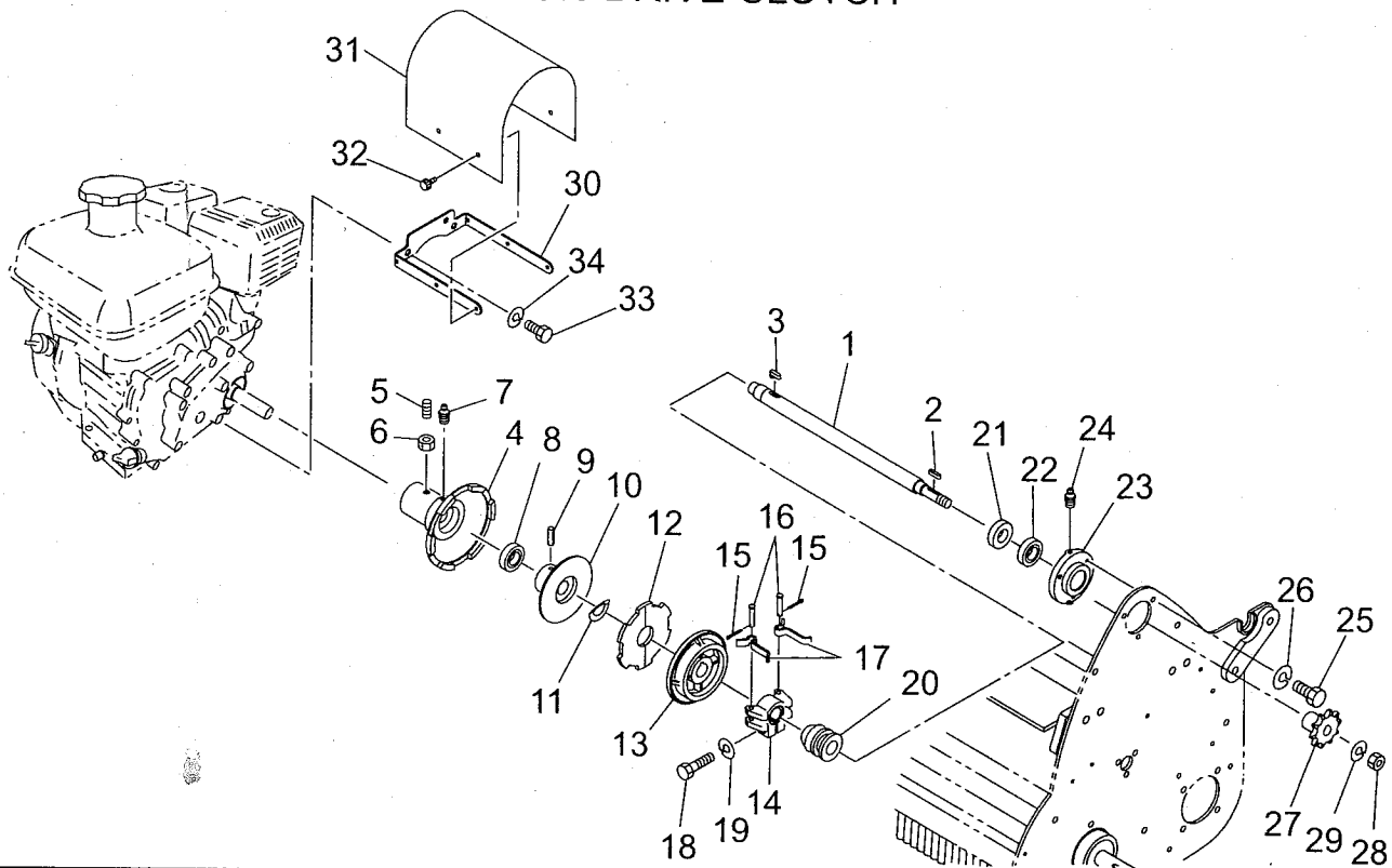
走行クラッチ FIG.6 DRIVE CLUTCH
