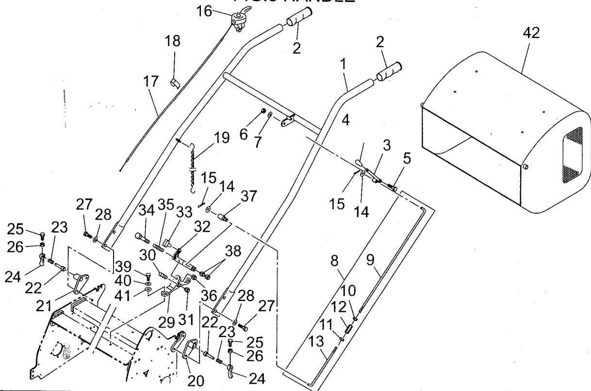
ハンドル FIG.8 HANDLE
