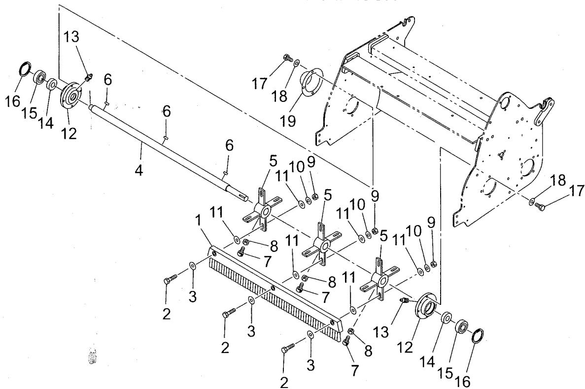
ブラシ FIG.5 BRUSH
