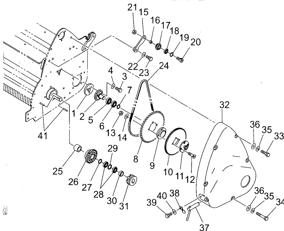
ブラシ駆動部 FIG.4 BRUSH DRIVE
