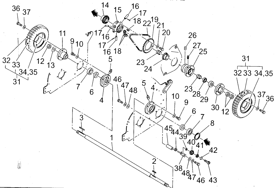
走行駆動部 FIG.7 TRAVELLING DRIVE
