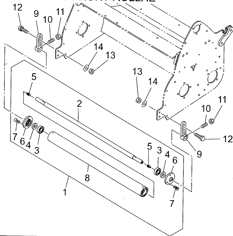
前ローラー FIG.3 FRONT ROLLRE
