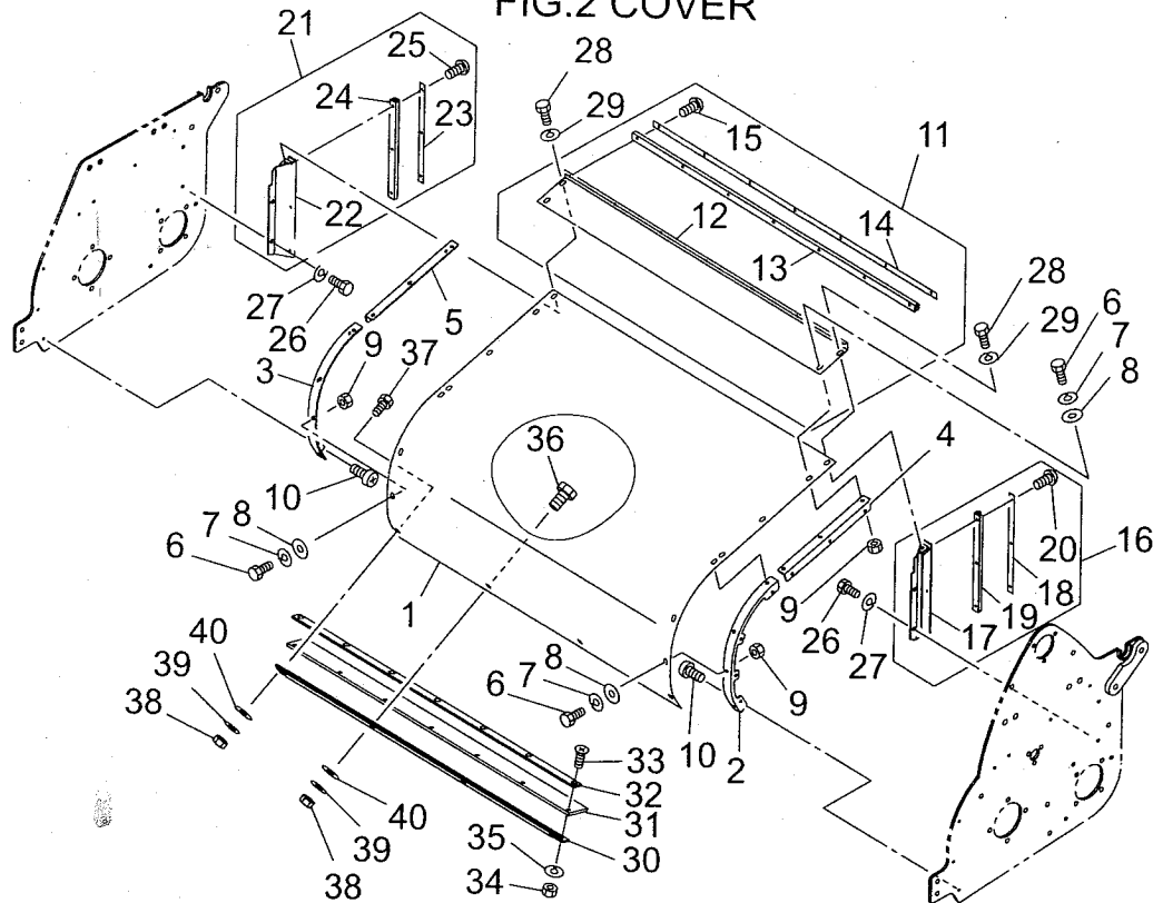
カバー FIG.2 COVER
