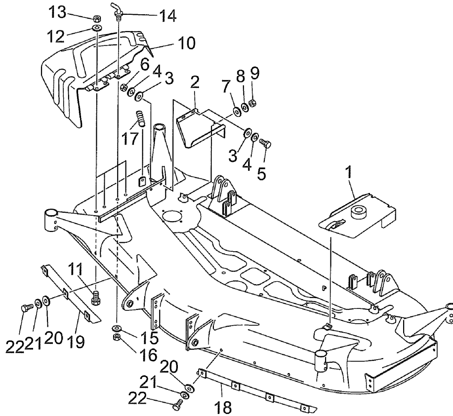
FIG.303 カバー COVER
