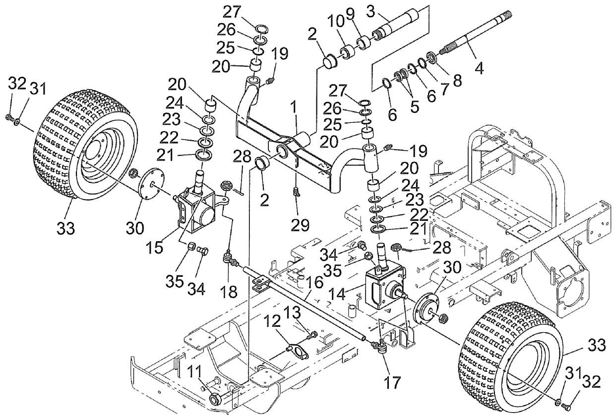
フロントアクスル FIG.206 FRONT AXLE
