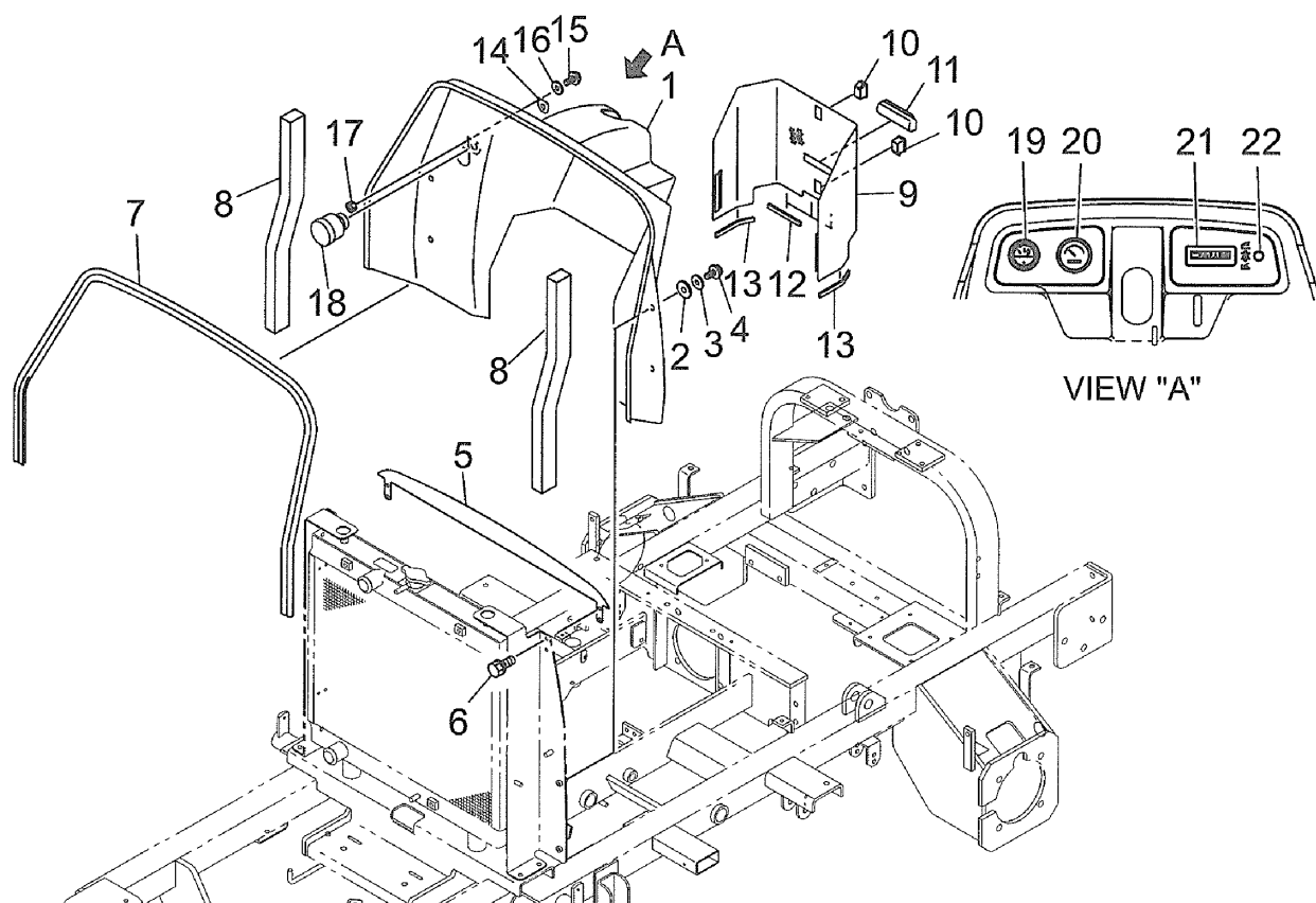
ダッシュボード FIG.212 DASH BOARD
