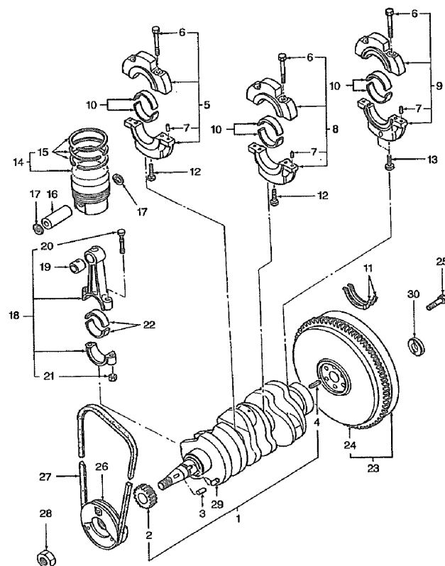
FIG.104 クランクシャフト、ピストン CRANKSHAFT,PISTON
