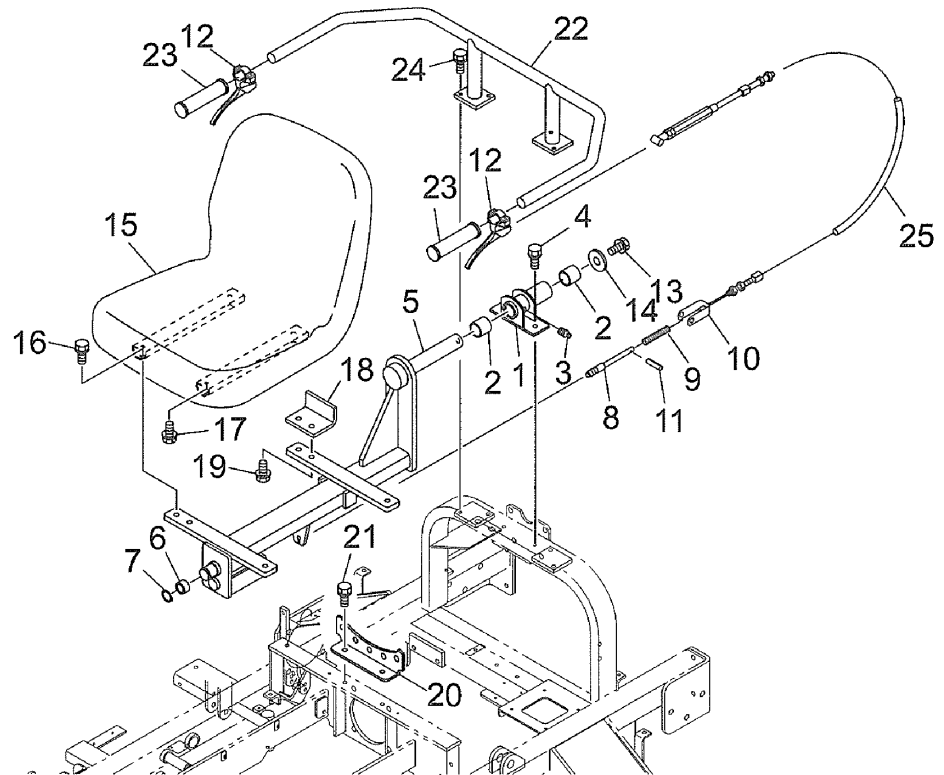
シート FIG.210 SEAT
