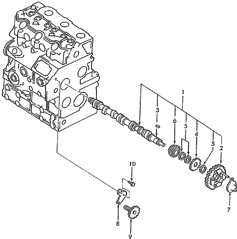
CAMSHAFT
