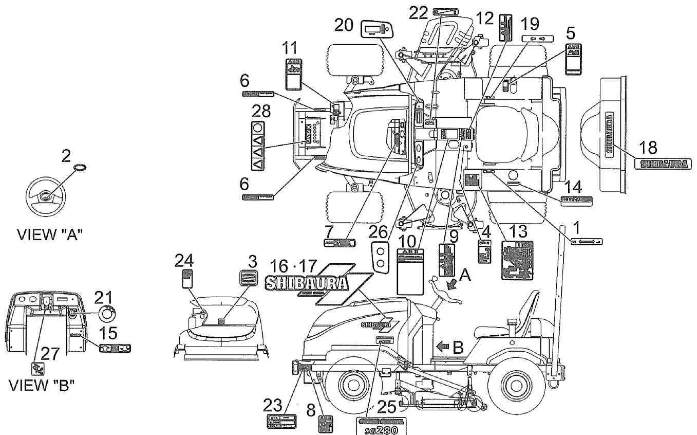
メイバン FIG.228 MARK
