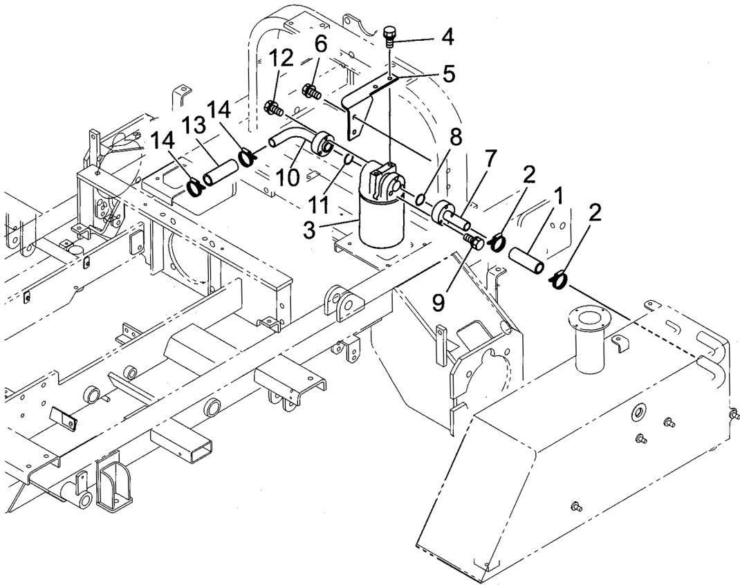
FIG.224 フィルタ FILTER
