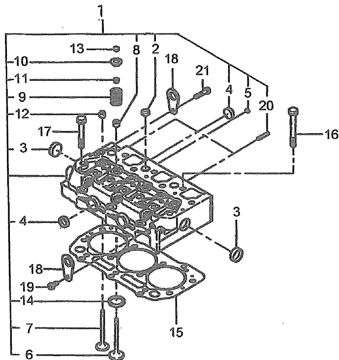
FIG.102 シリンダヘッド CLYINDER HEAD
