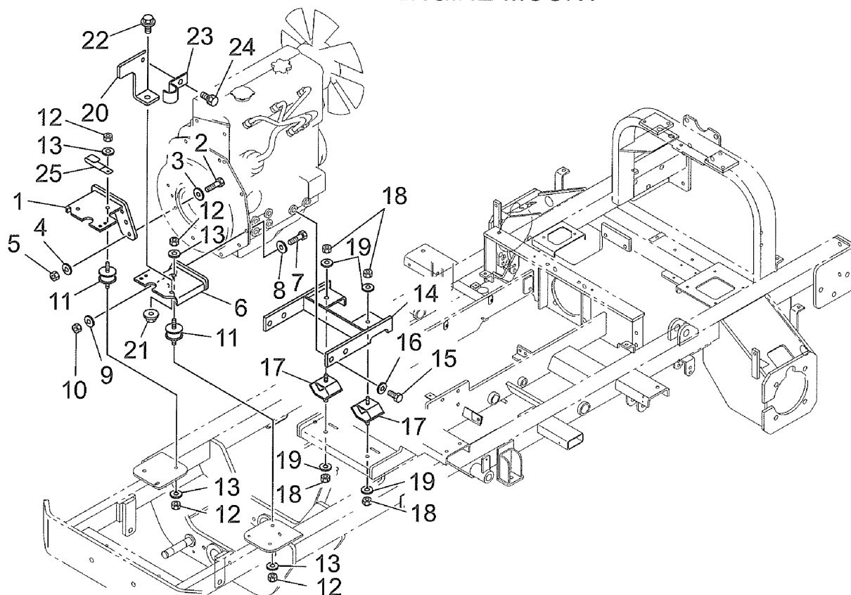
エンジンマウント FIG.204 ENGINE MOUNT
