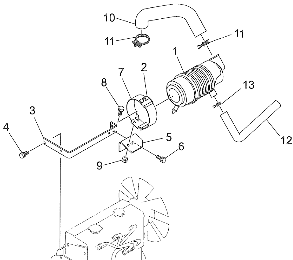
FIG.202 エアークリーナー AIR CLEANER
