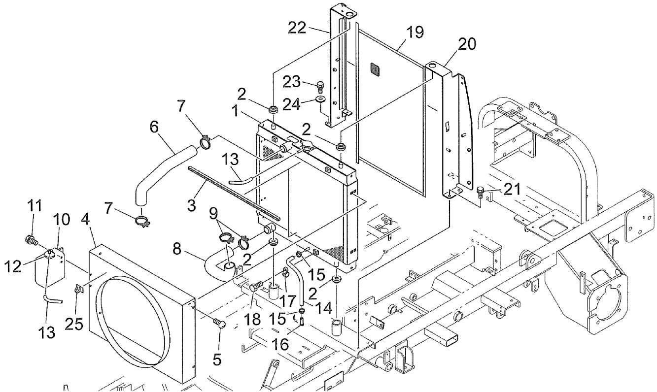
FIG.203 ラジエータ RADIATOR
