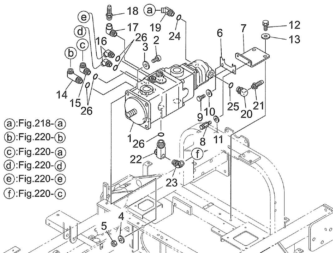
FIG.222 ユアツ(H.S.T) HYDRAULIC(H.S.T)
