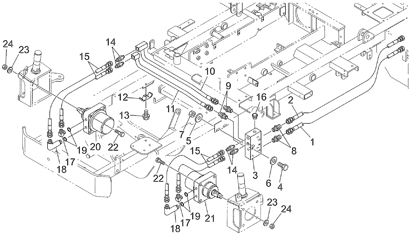
FIG.217 ユアツ (フロントソウコウ) HYDRAULIC(FRONT AXLE)
