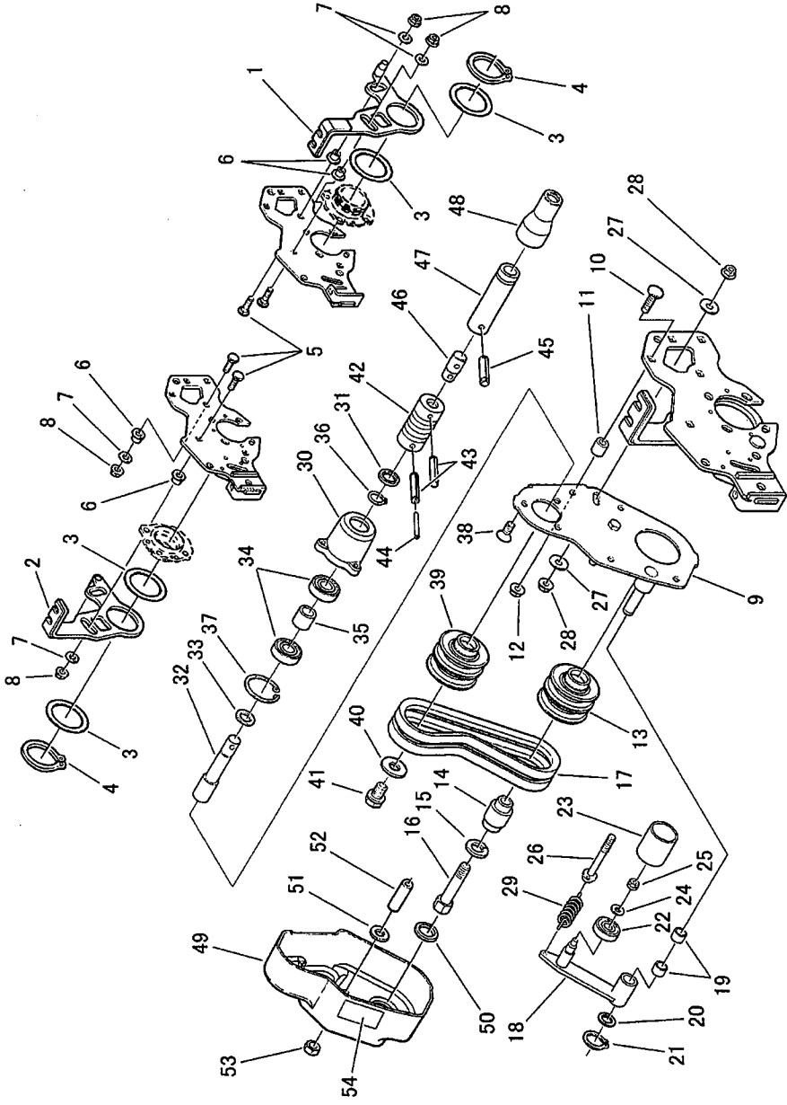
ARM-CLUTCH
