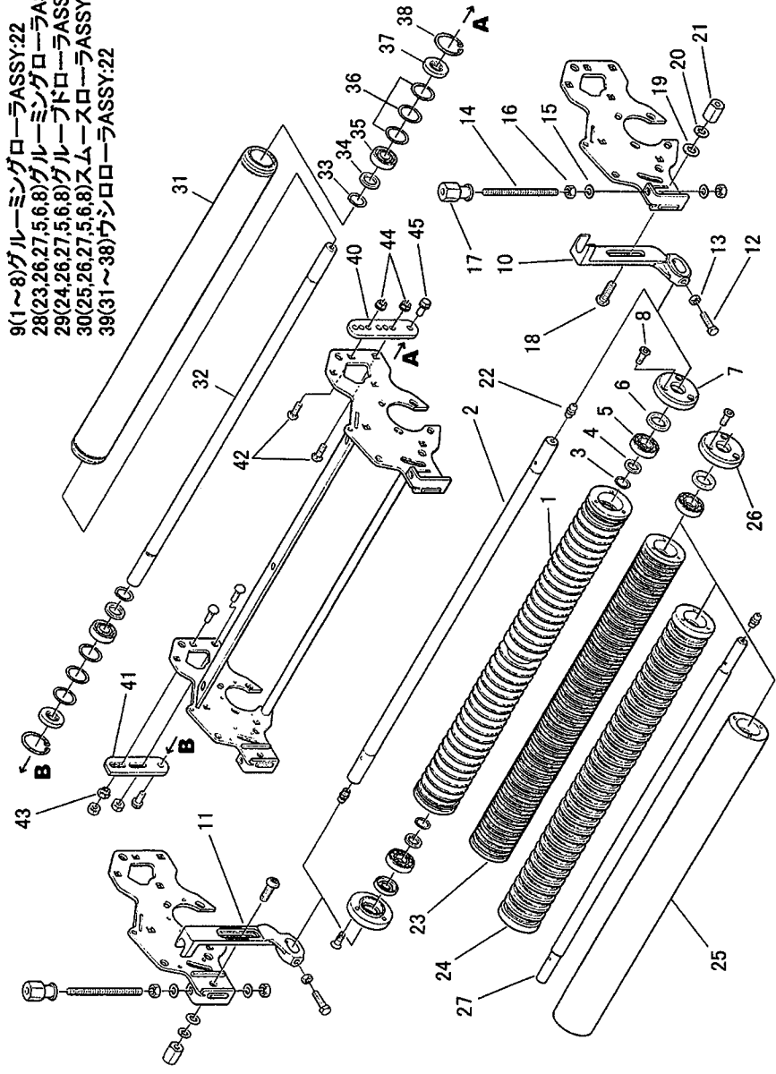
前後ローラ関係 FIG. 11 FRONT/REAR ROLLER
